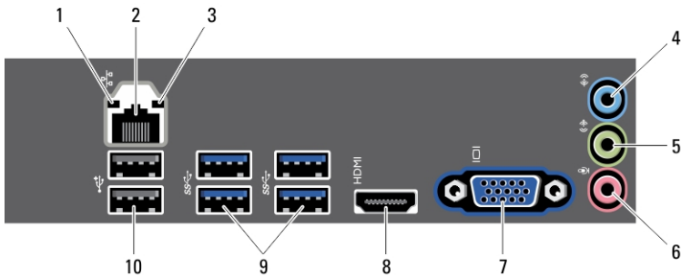
Afbeelding 2. Aanzicht van achterpaneel
